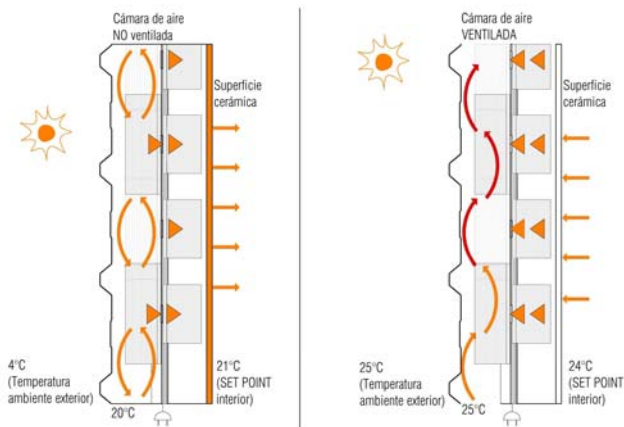
Figura 3: Esquema del comportamiento energético de la fachada activa termoeléctrica con los disipadores interio durante régimen de invierno (a) y verano (b).
